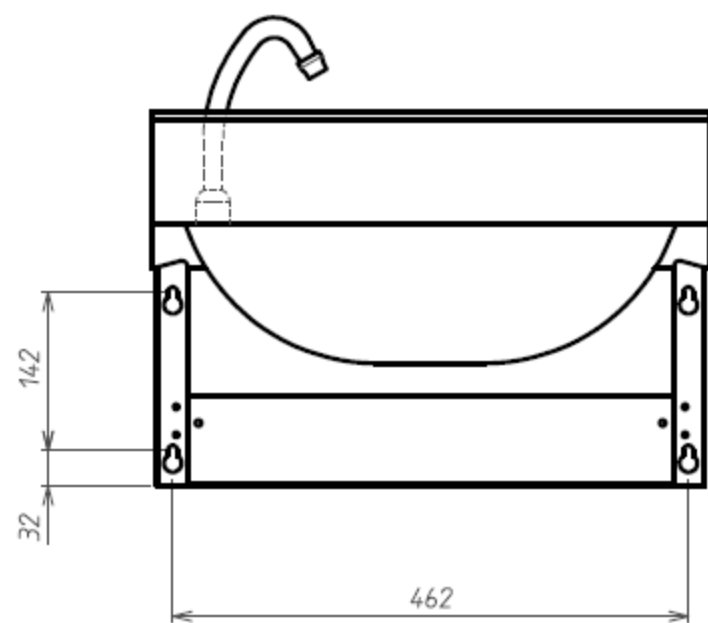
vista posteriore
