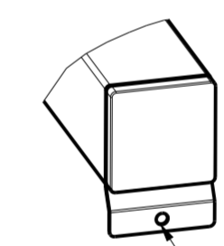
B(2:5) FORO FISSAGGIO D4.5 FIXING HOLE D4.5
